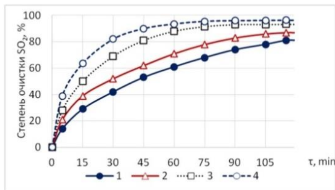
Рисунок 3 – Влияние содержания \text{CO}_2 в газовой смеси на степень очистки с применением аммония гидроксида: C_{\text{NH}_4\text{OH}} = 5 \div 10\% , C_{\text{SO}_2} = 26 \div 85 . 1 – C_{\text{SO}_2} = 0,85\% ; 2 – C_{\text{SO}_2} = 0,65\% ; 3 –
