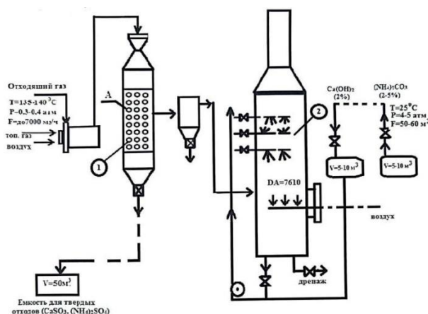
Рисунок 1 – Принципиальная технологическая схема усовершенствования установки очистки дымовых газов. Где: А – сухой очистка отходящих газов новым адсорбентом (ТХТИ). 1-Скуббер сухой очистки; 2-Скуббер колонна мокрой очистки
